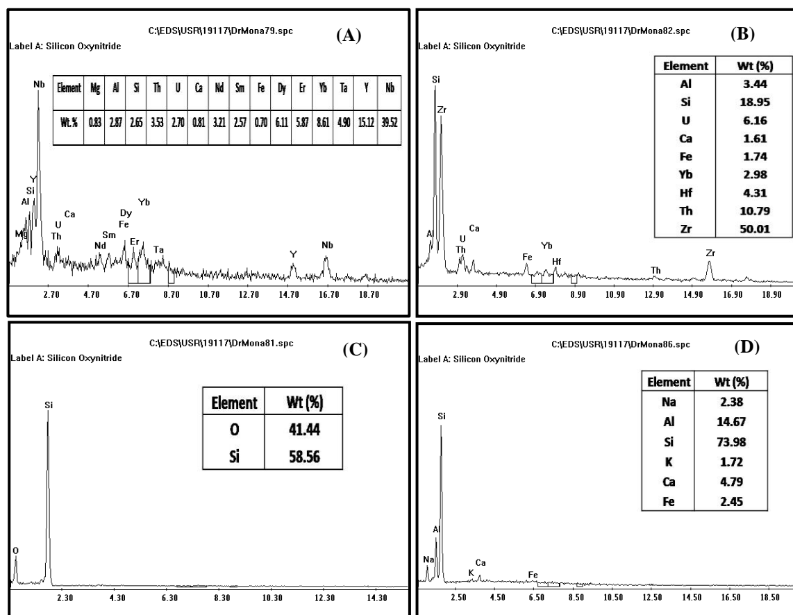
Fig. 1. EDX analysis data of fergusonite (A), zircon (B), quartz (C), and feldspar (D)
