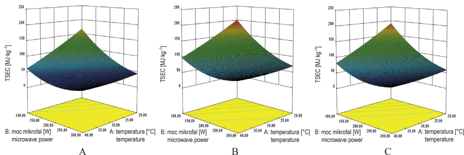
Rys. 2. Płaszczyzna odpowiedzi całkowitego właściwego zużycia energii TSEC do MR = 0,02 w zależności od temperatury (czynniki A) i mocy mikrofal (czynniki B) otrzymana w przypadku liści pietruszki poddanych ultradźwiękom (A), obróbce parą wodną (B) i moczeniu (C)
