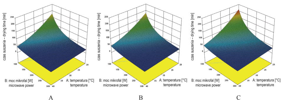
Rys. 1. Płaszczyzna odpowiedzi czasu suszenia do MR = 0,02 w zależności od temperatury (czynniki A) i mocy mikrofal (czynniki B) otrzymana w przypadku liści pietruszki poddanych ultradźwiękom (A), obróbce parą wodną (B) i moczeniu (C)
